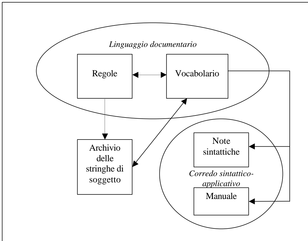
Fig. 1: Componenti del Sistema Nuovo Soggettario e loro relazioni
