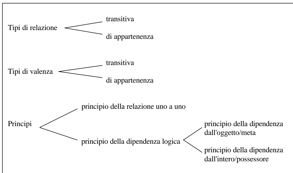
Fig. 6: Carattere dualistico del modello sintattico
